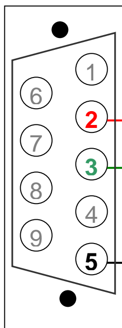
Poz. 1. Pogled sa strane lemljenja
